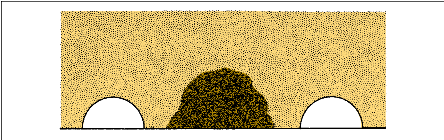
Fig. 6: Lille lagtykkelse i forhold til kanalafstand øger risikoen for dårlig fordeling af tørreluften
